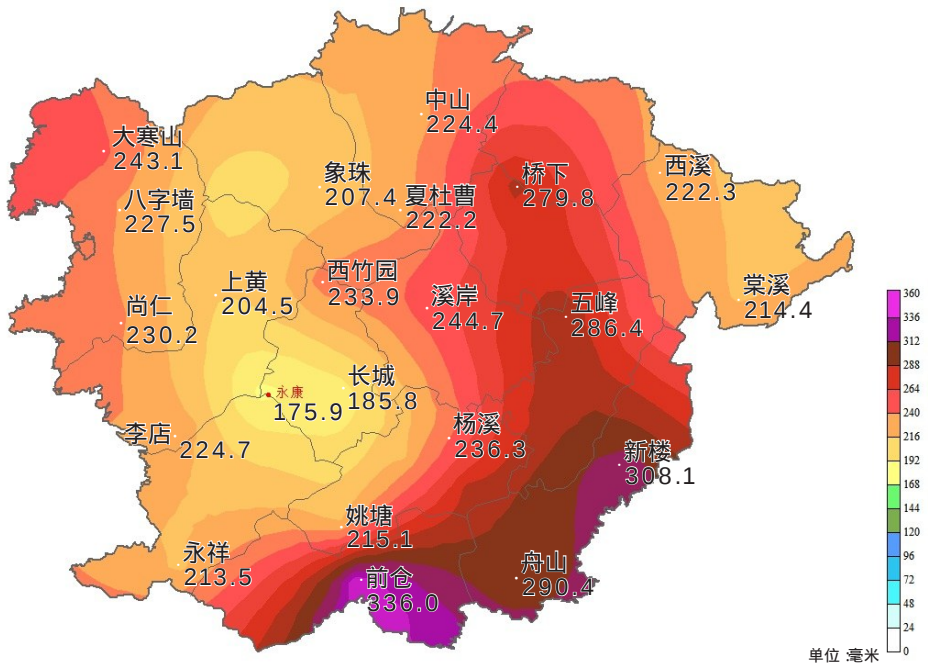
6月9日20时至7月4日20时全市累积雨量分布图
